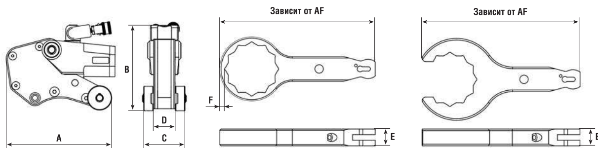
Привод с картриджем
